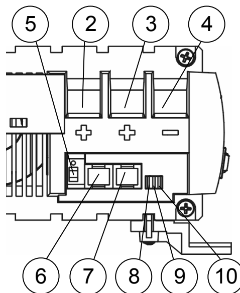
Figura 2: Conexiones
