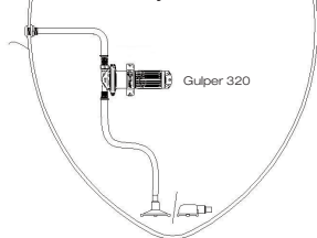
Instalación típica como bomba de achique de montaje remoto
