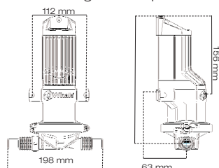
Typisk installation som avloppspump med hög kapacitet
