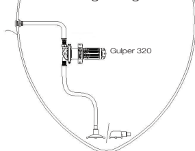
Installation typique de pompe de cale à montage éloigné
