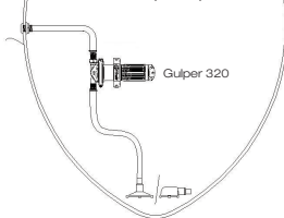
Typische Installation als ferninstallierte Lenzpumpe
