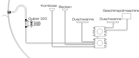
Typische Installation als ferninstallierte Lenzpumpe
