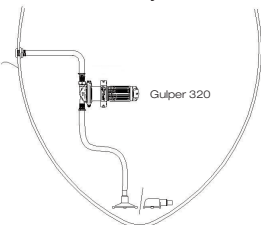
Typisk installation som fjärrmonterad länspump
