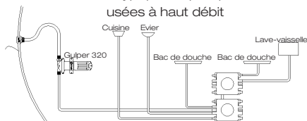
Installation typique de pompe à eaux usées à haut débit
