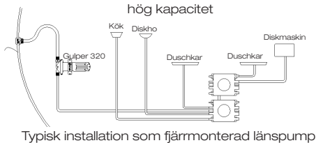
Typisk installation som fjärrmonterad länspump
